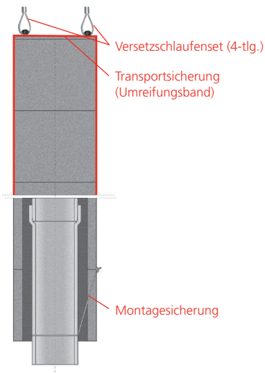
Bild 3: Überdruckabgasleitung SÜ
