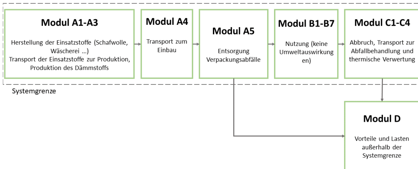
Abbildung 3: Flussdiagramm Lebenszyklusphasen
