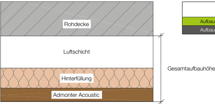
AUFBAU
