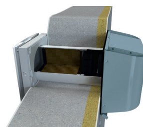
Montagebeispiel mit der Haube für dünne Wände AH-S grey 160 / AH-S chrome 160
