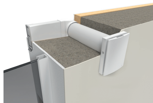
Laibungskit in einer Wand mit üblicher Wandstärke mittels des Montagesatzes KIT BlauPlast white 160 / KIT BlauPlast chrome 160
