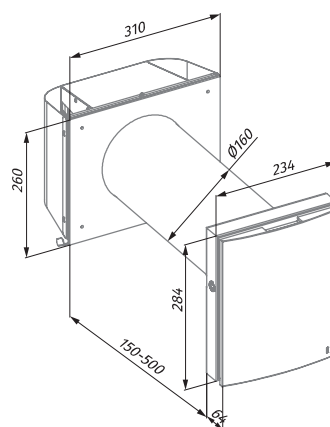
VENTO Expert A50-1 S Pro (für dünne Wände)
