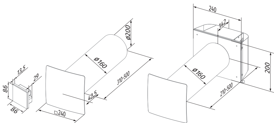
VENTO ECO2 A50 S10 Pro
