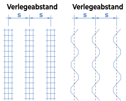
Draufsicht Verlegeschema bei Körben:
