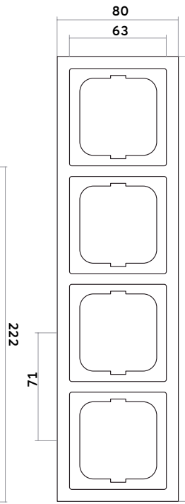
Abdeckrahmen 4-fach
