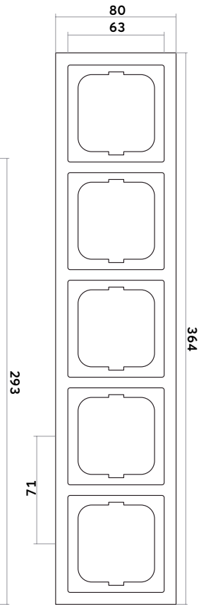
Abdeckrahmen 5-fach
