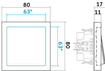
Schalter
