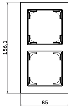
Abdeckrahmen 2-fach
