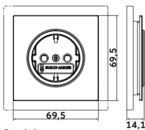
Steckdose
