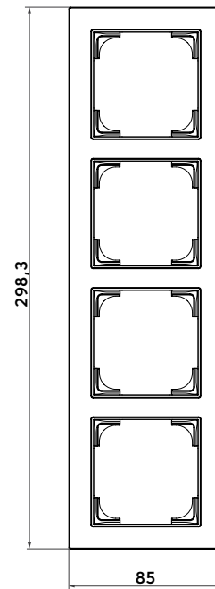
Abdeckrahmen 4-fach
