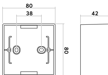
AP-Gehäuse 1-fach
