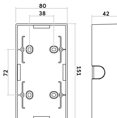
AP-Gehäuse 2-fach
