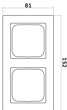
Abdeckrahmen 2-fach
