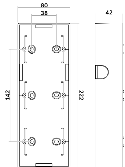
AP-Gehäuse 3-fach
