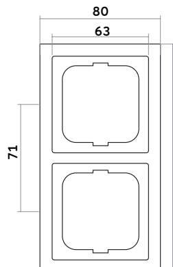
Abdeckrahmen 2-fach
