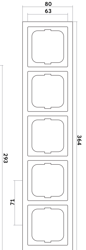
Abdeckrahmen 5-fach
