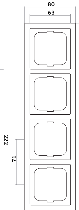
Abdeckrahmen 4-fach
