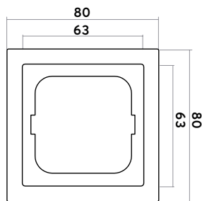
Abdeckrahmen 1-fach
