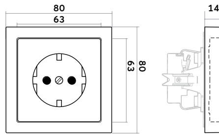
Steckdose
