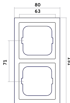
Abdeckrahmen 2-fach
