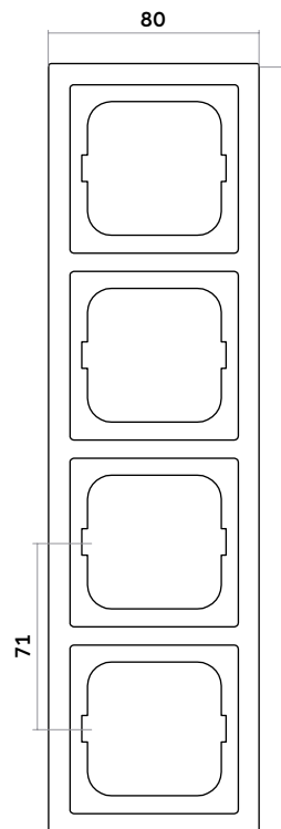
Abdeckrahmen 4-fach
