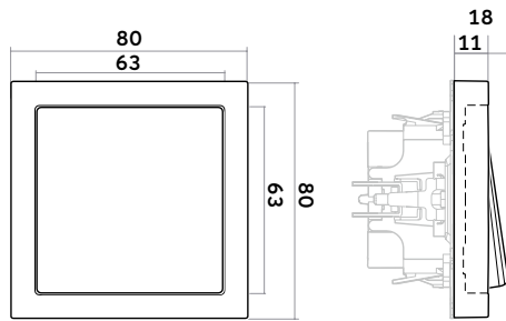
Schalter
