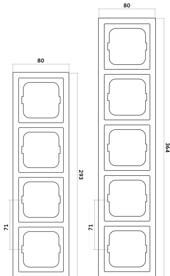
Abdeckrahmen 5-fach
