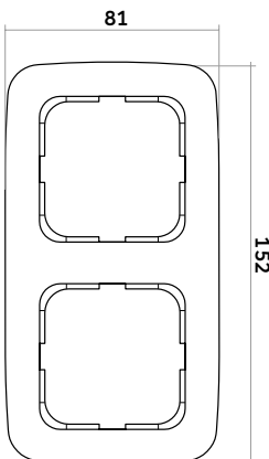
Abdeckrahmen 2-fach
