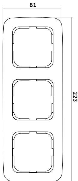
Abdeckrahmen 3-fach
