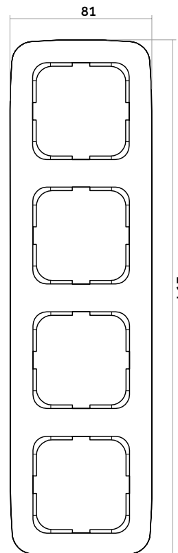
Abdeckrahmen 4-fach
