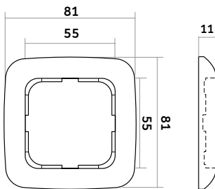
Abdeckrahmen 1-fach
