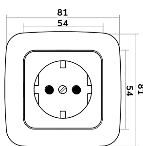
Steckdose
