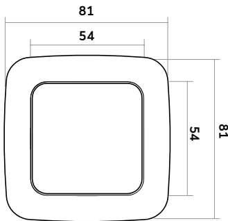
Schalter
