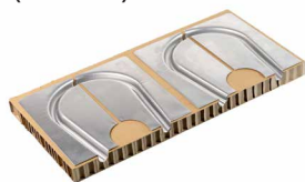
EQ Decken-/Wandmodul LIGHT Alu-Umlenkelement (2 Bögen – geteilt) 250 x 500 x 30 mm (L x B x H)
