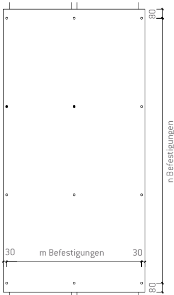
vertikale Tafelanordnung
