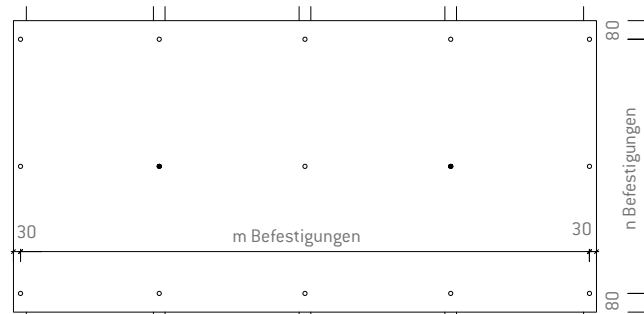
horizontale Tafelanordnung
