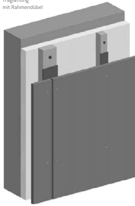
Holz-Unterkonstruktion mit Abstandhaltern
