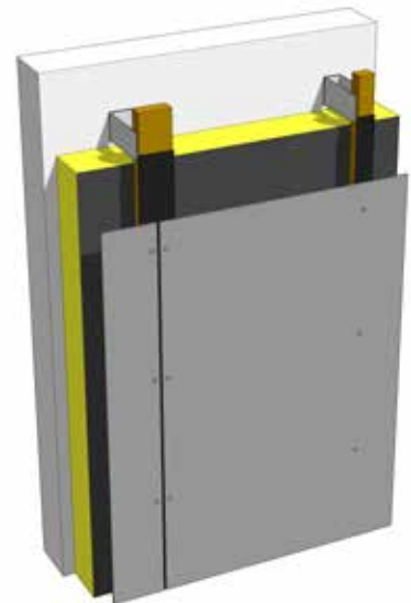
Holz-Unterkonstruktion mit Abstandhaltern
