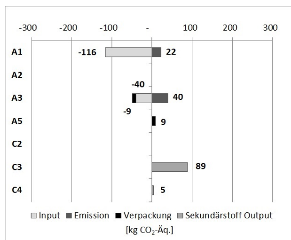
Abb. 3: Holzinhärente CO 2 -Produktsystemein- und -ausgänge [kg CO 2 -Äq.]. Die inverse Vorzeichengebung der In- und Outputs trägt der ökobilanziellen CO 2 -Flussbetrachtung aus Sicht der Atmosphäre Rechnung.
