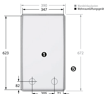
Frontansicht (Längenangaben in mm)
