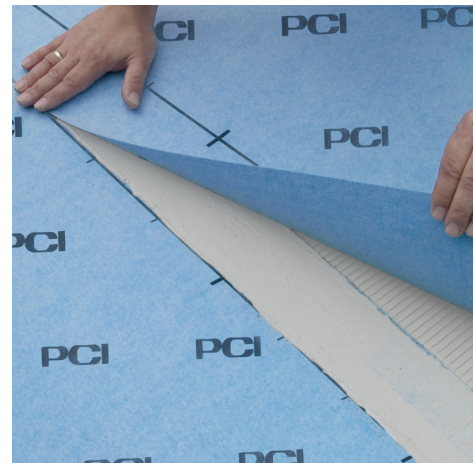
PCI Pecilastic Roll&Go härtet sicher unter den Überlappungen der Abdichtungsbahn PCI Pecilastic W aus.
