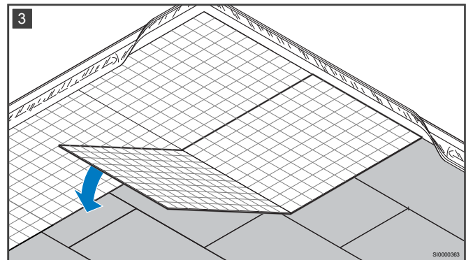
3 Uponor Klett Twinboard Panels verlegen
