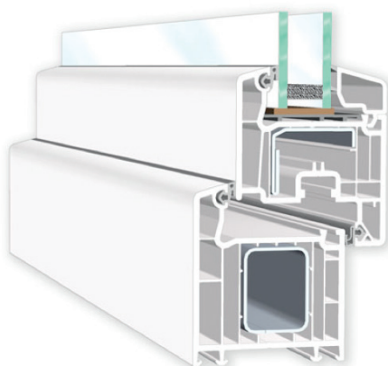
SOFTLINE (Flügel flächenversetzt)
