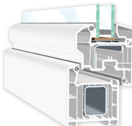
SOFTLINE (Flügel halbflächenversetzt)
