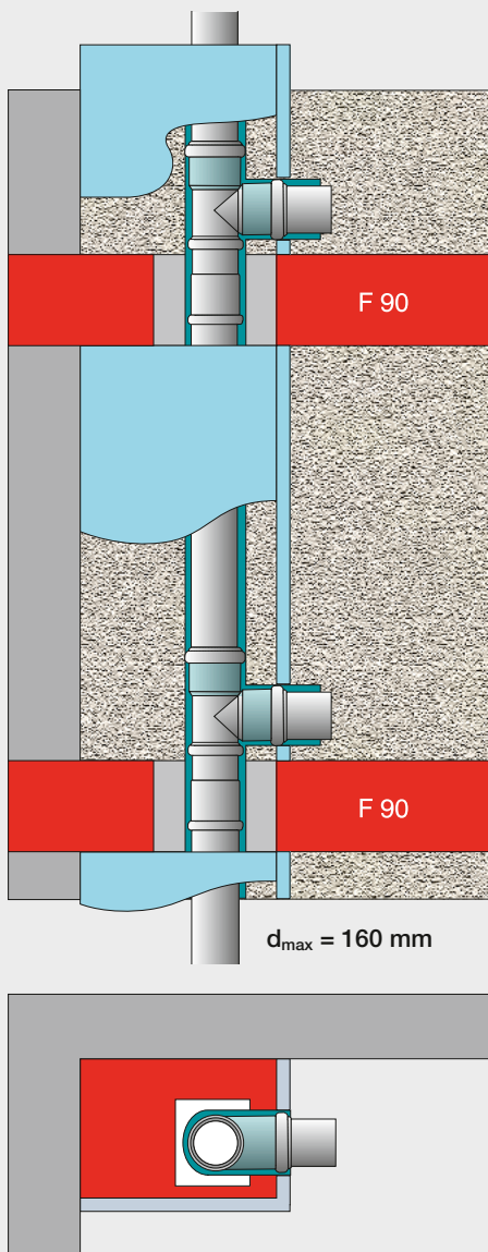
Abb. 30: Schachtinstallation (Vorwandsystem)
