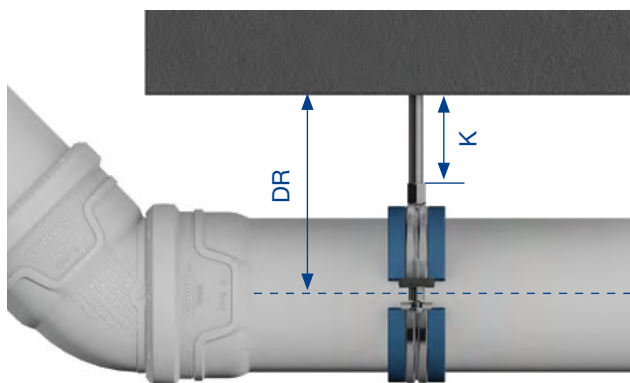
Horizontaler Abstand von der Rohrschelle zum Mauerwerk
