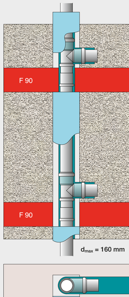
Abb. 31: Unterputzinstallation (Mauerschlitz)
