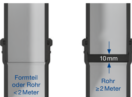
Abb. 44: Berücksichtigung von Längenänderungen bei Steckverbindungen
