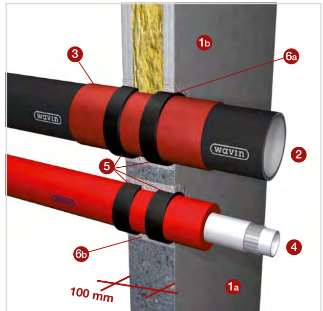
Bild 2: Gerade Rohrführung durch Wand.
