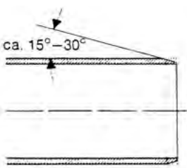
Abb. 53: Einschubende anschrägen
