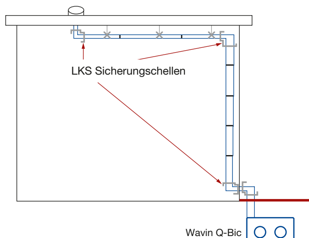
Abb. 37: Montageschritte Wavin LKS-Schelle
