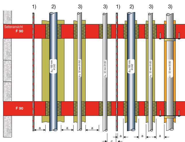
Abb. 28: Einzelne Rohrleitungen mit Dämmung in Durchbrüchen oder Kernbohrungen
