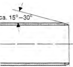
Abb. 53: Einschubende anschrägen
