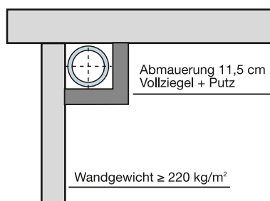
Abb. 47: Innenliegende Regenfallleitung
