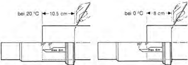
Abb. 55: Einschublänge in Abhängigkeit von der Montagetemperatur
