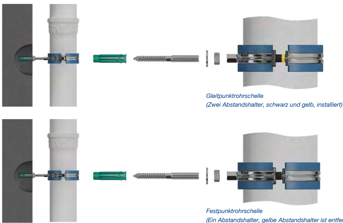
Abb. 42: Wavin Schallschutzrohrschelle
