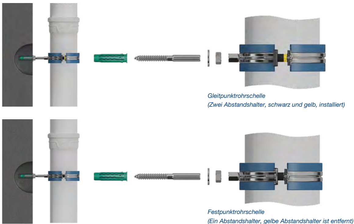
Abb. 42: Wavin Schallschutzrohrschelle
