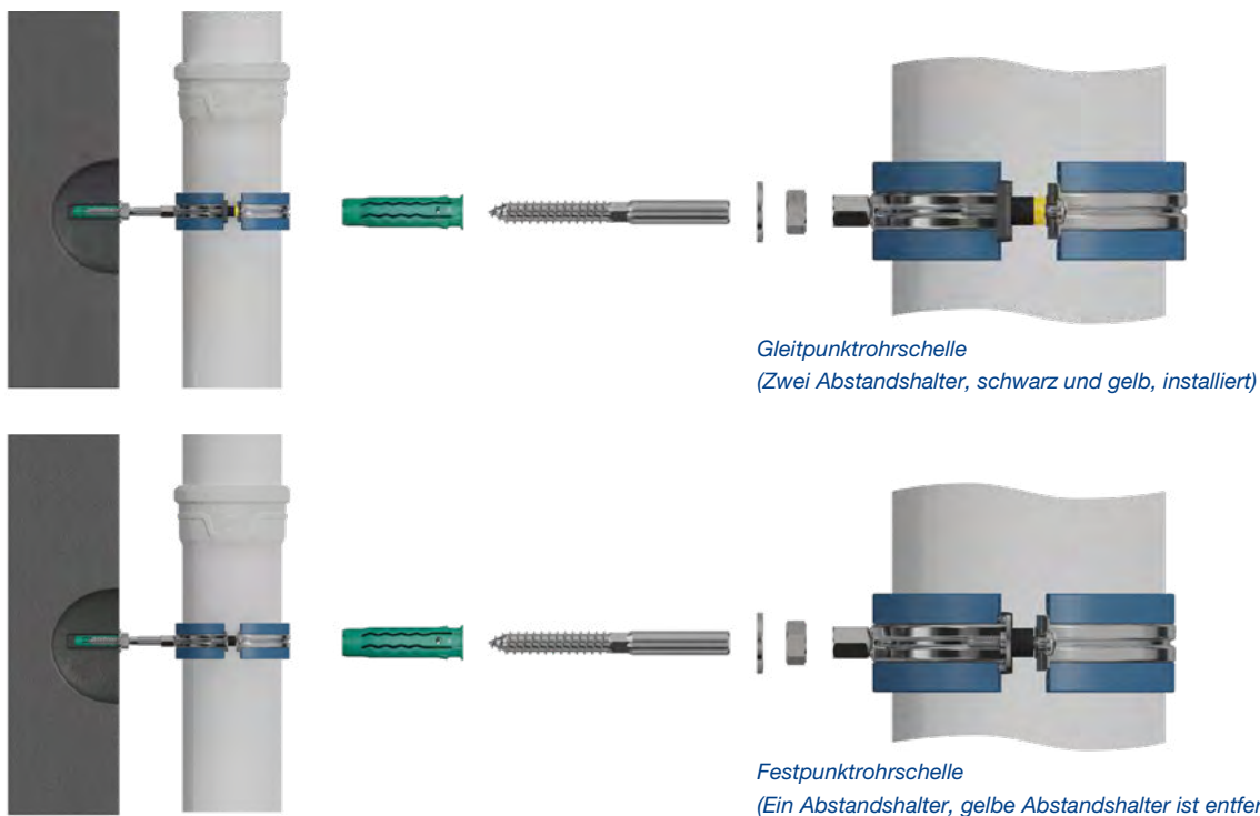
Abb. 42: Wavin Schallschutzrohrschelle
