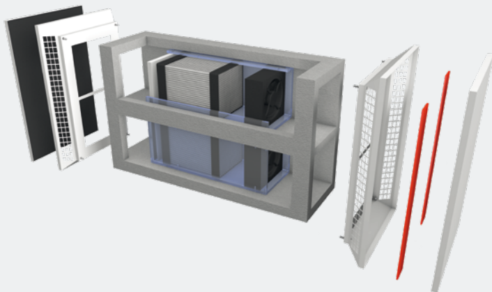
AIRUNIT GEMINI Dezentrale Wohnraumlüftung Art.-Nr. 4 02 011
