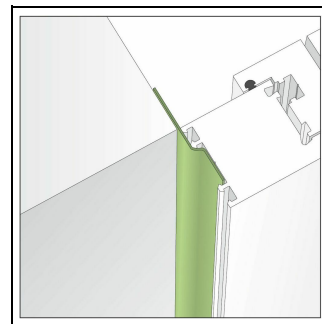
4. Bild: Folie auf die Außenseite des Blendrahmens kleben, Folie in der Flucht zur Wandaufbahrung führen
